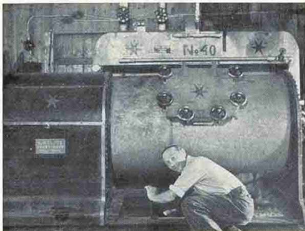
Maskin för kemisk tvätt. Fabrikat Lind- sjö, Trelleborg.
